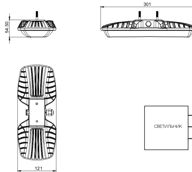
Рисунок 1. Габаритный чертеж
